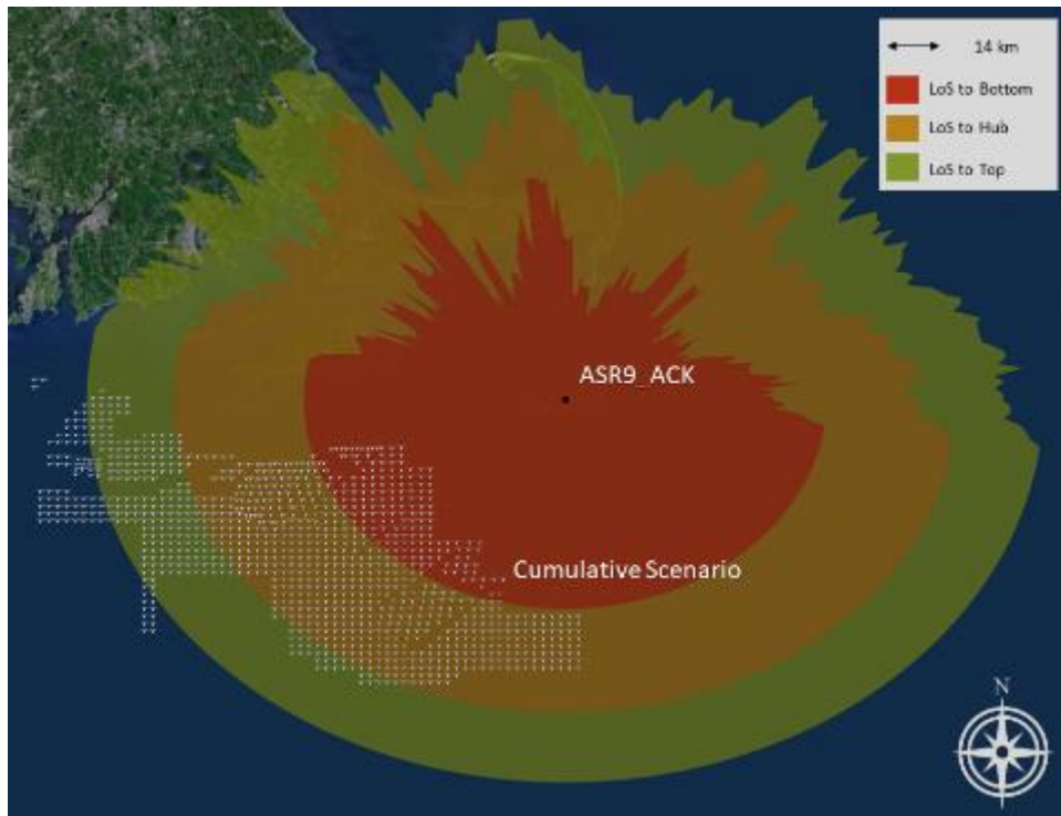
Figure 224 - RI/MA Cumulative Scenario, ASR-9, ACK
